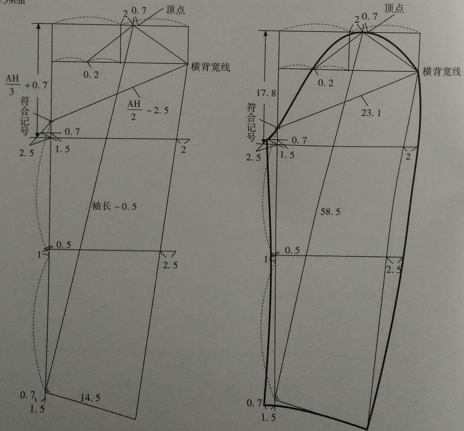
步骤 5: 测量衣身袖窿弧线长度 AH = 51.2cm
