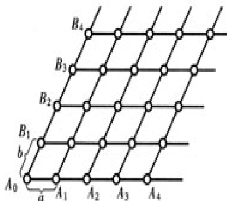
图 2-5 面网
