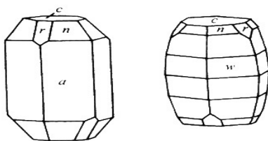
图 10-2 刚玉的晶体
