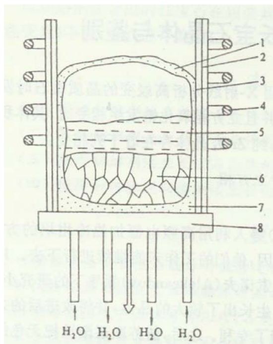
1.熔壳盖 2.石英管 3.水冷用铜管 4.高频线圈（RF） 5.熔体 6.晶体 7.未熔料 8.水冷座
